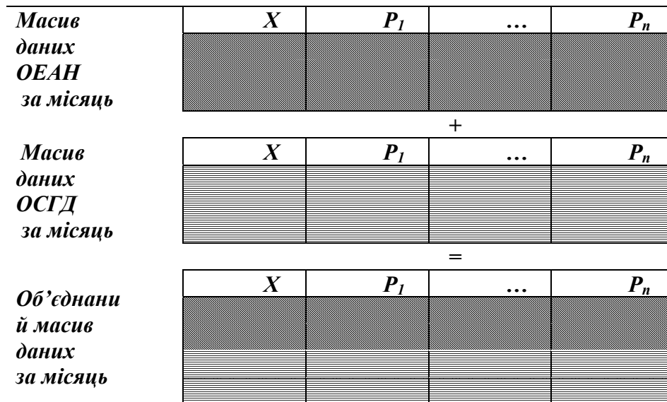
Рис. 3. Схема об'єднання щомісячних даних ОЕАН за основною вибіркою та за вибіркою ОСГД в єдиний масив
